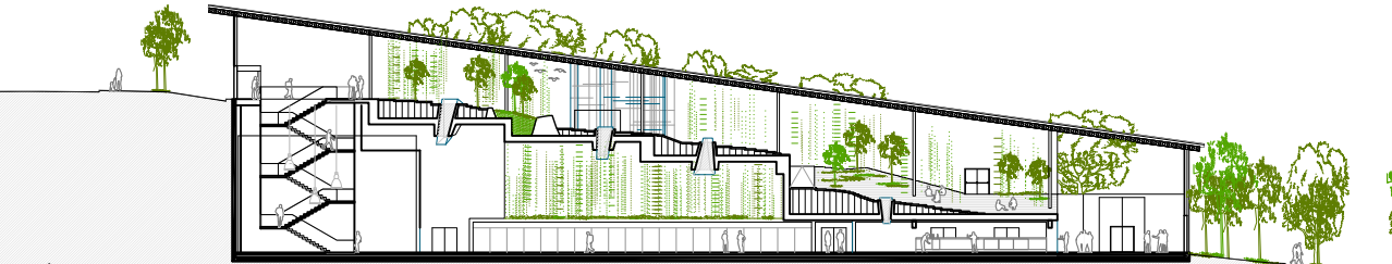
SECCIÓN LONGITUDINAL POR DISTRIBUIDOR
