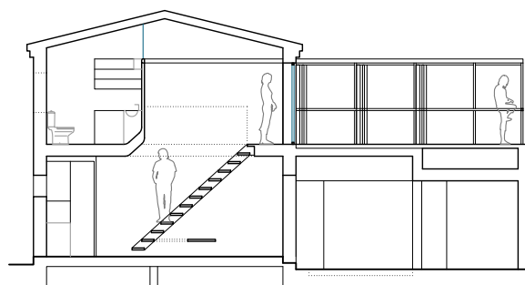
SECCIÓN LONGITUDINAL POR ESCALERA
