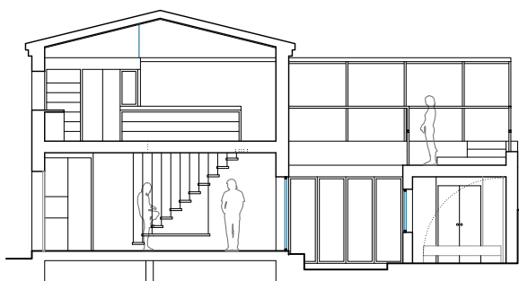
SECCIÓN LONGITUDINAL POR PATIO
