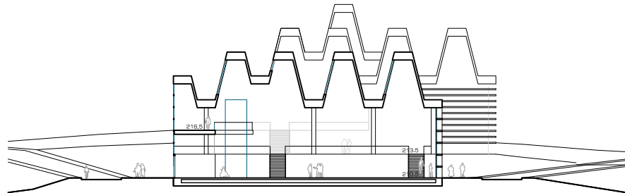
SECCIÓN TRANSVERSAL
